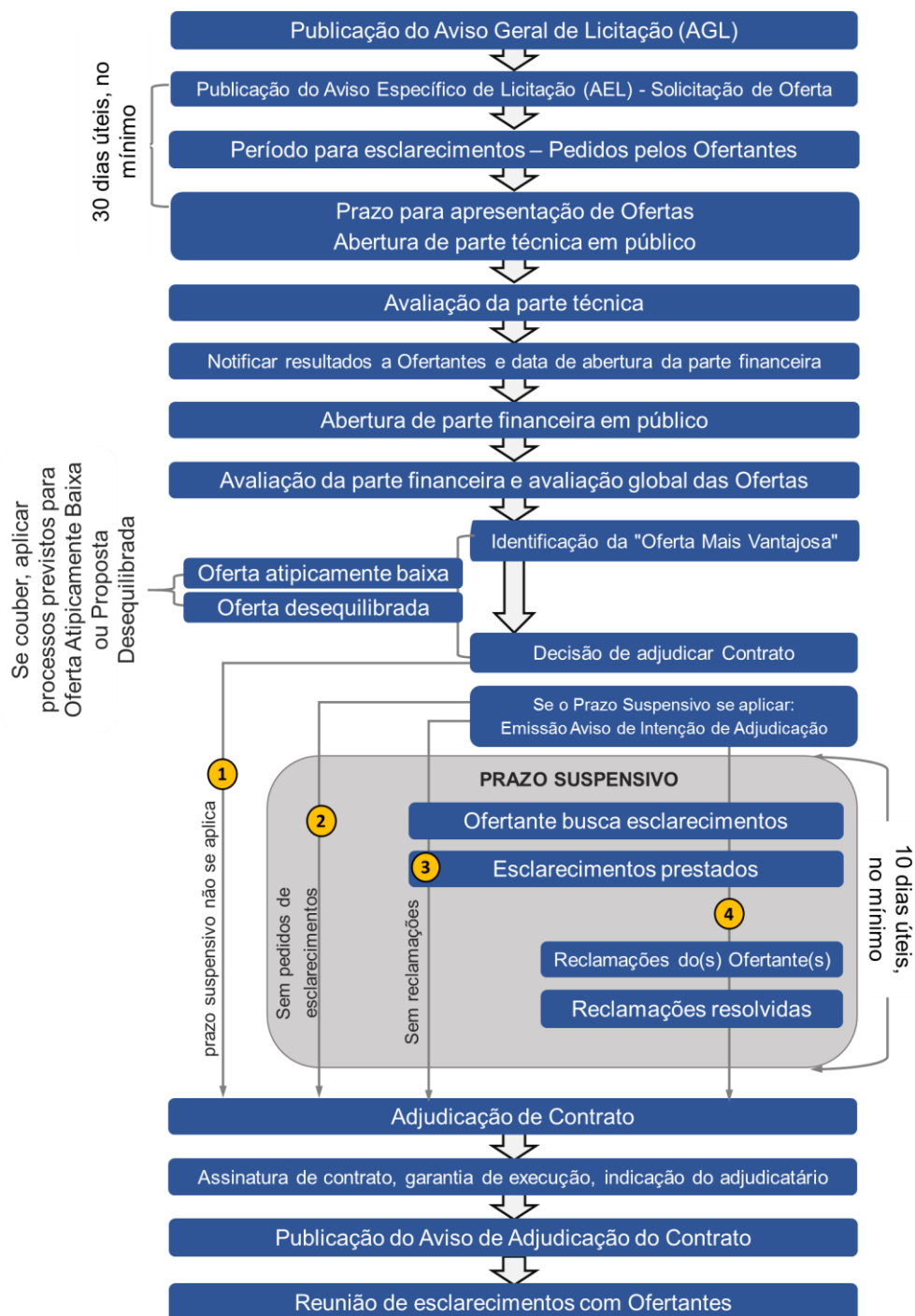
Figura 7: Fluxograma de processo: SDO no processo com dois envelopes (sem Pré-qualificação)
