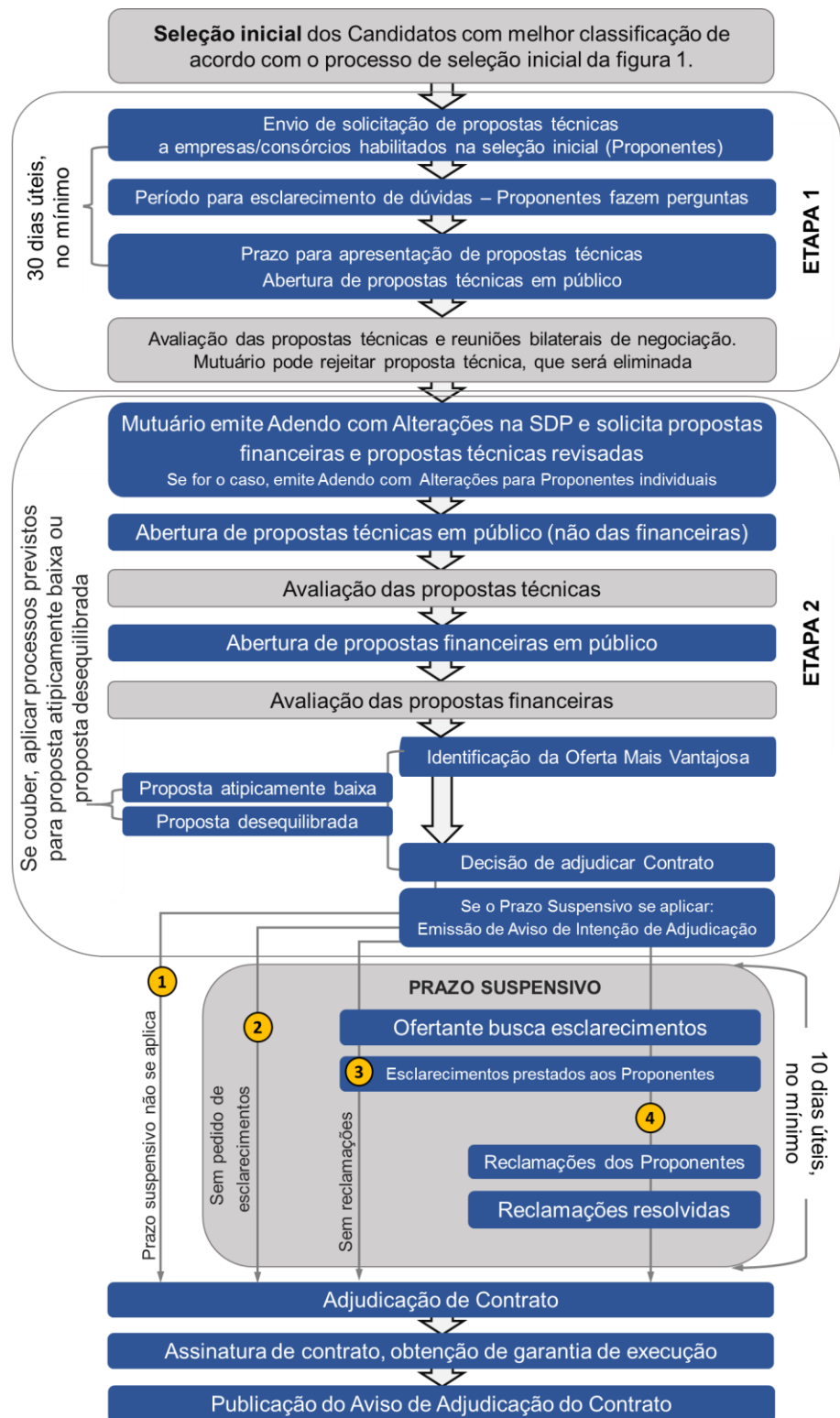
Figura 2: Fluxograma de processo: SDP - Modelo 1
